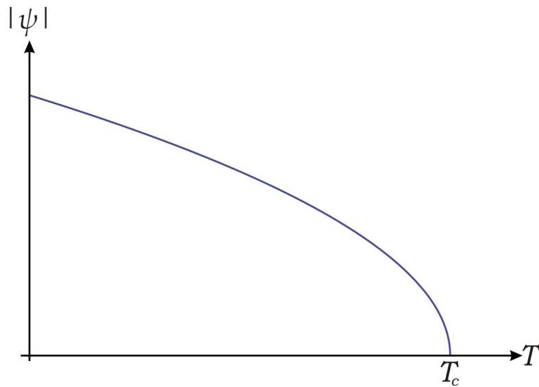
Figura 3.3: Gráfico do módulo do parâmetro de ordem com relação à temperatura. Queda abrupta da função quando T \rightarrow T_c
