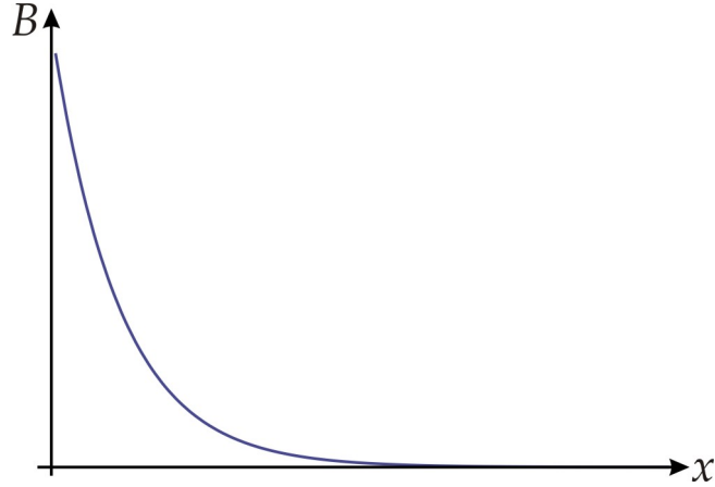
Figura 2.7: Dependência do campo magnético com a distância no interior da amostra
