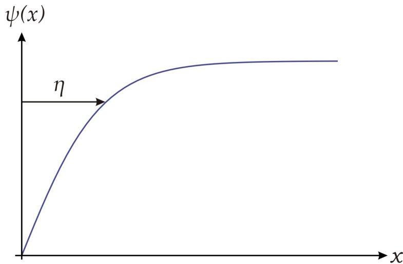
Figura 3.4: O parâmetro de ordem de um supercondutor próximo à sua superfície. A recobrada do valor \psi_o ao longo do comprimento de coerência \eta(T) .
